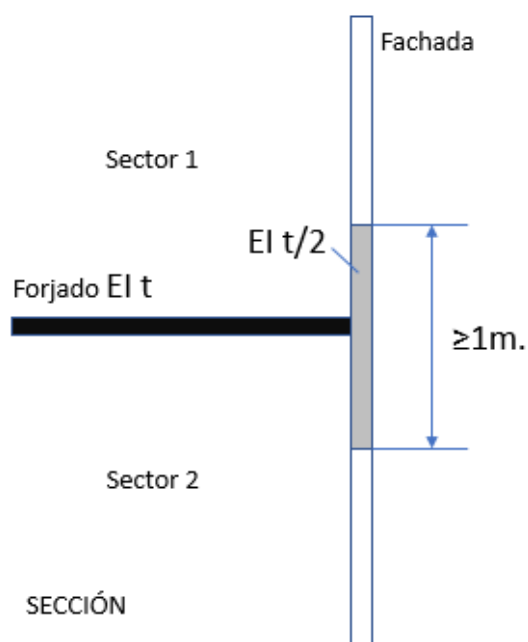
Figura 2.9: Compartimentación vertical.
